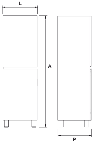
Coluna Tipo 2 Column Type 2
