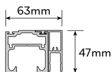
Perfil parede Wall profile Profil mural
