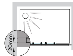
Aplicação a partir do rebordo da base Application from the edge of the base
