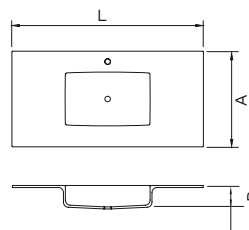
Lavatório Cerâmico. Ceramic washbasin
