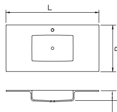
Lavatório Cerâmico. Ceramic washbasin
