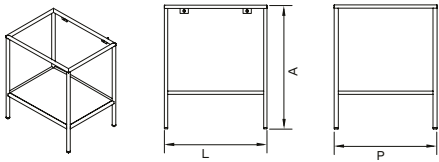
Estrutura lavatório de encastrar Built-in washbasin frame
