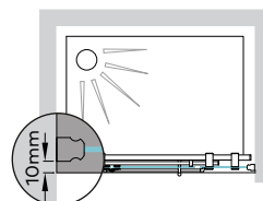
Aplicação a 10mm do rebordo da base Application 10mm edge of the base
