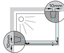
Aplicação a 10mm do rebordo da base Application 10mm edge of the base
